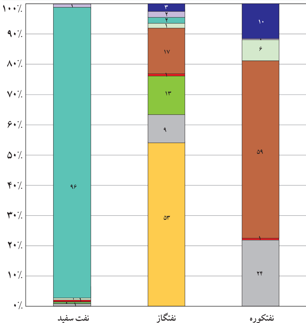
نمودار درصد مصرف نفت سفید نفتگاز و نفتکوره در بخش‌های مختلف مصرف در سال ۱۳۸۸
